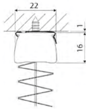
Потолочный
