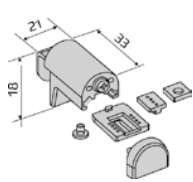
Кронштейн ПВХ
