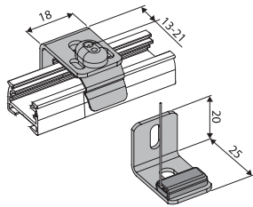
Стеновой стандартный
