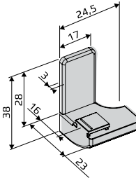
Стеновой закрытый
