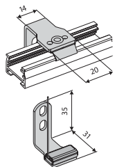
Стеновой стандартный
